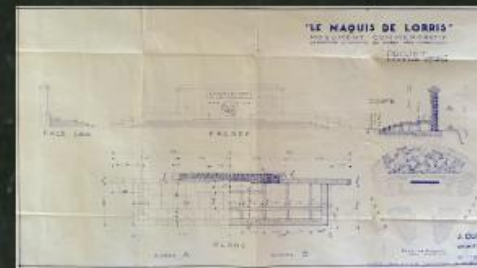
Projet du monument commémoratif par J. Cury, architecte à Montargis, 13 décembre 1944
